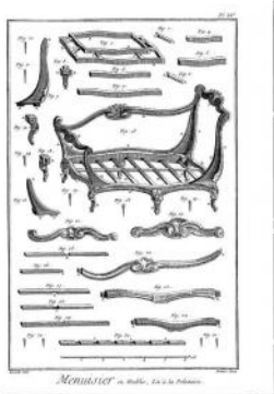
Menuiserie en Noix, Sa à la Polonoise
